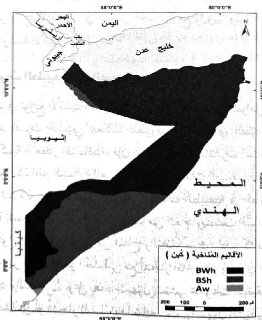
شكل (٩) الأقاليم المناخية في الصومال تبعاً لتصنيف كبن للمناخ
