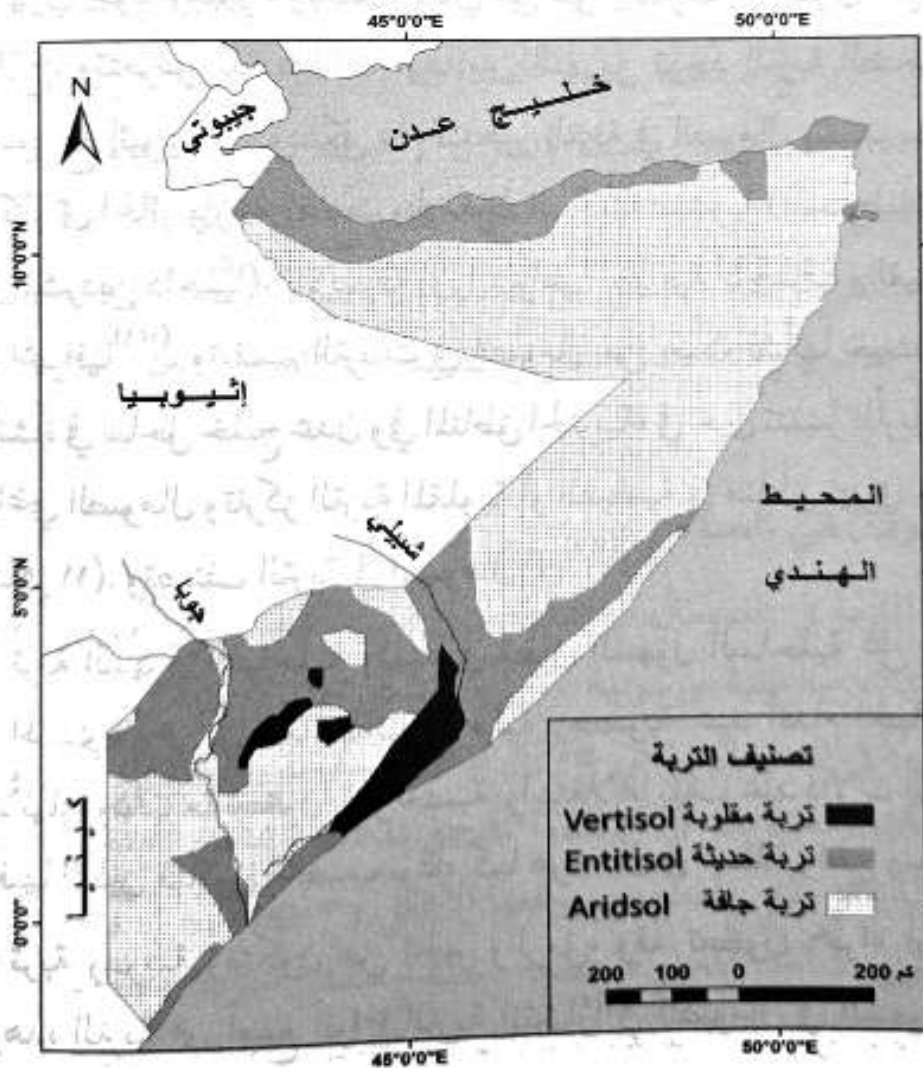
شكل (١١) التربة في الصومال
