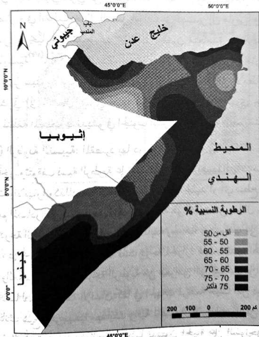
شكل (٨) التوزيع السنوي للرطوبة النسبية في الصومال
